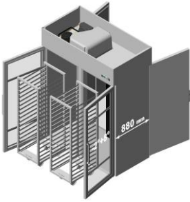
Indbygget kompressor J170/4MV2 J121702005
